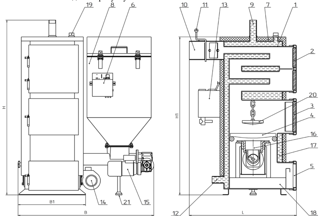
Рисунок 1 – Зовнішній вигляд та основні елементи котла типу КТ-2Е-ш
